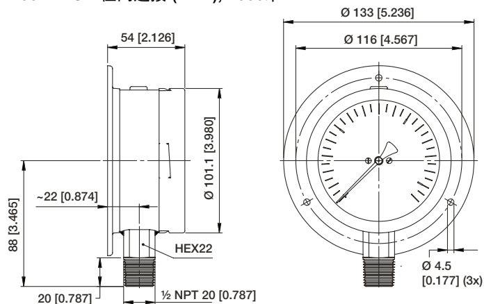
100mm SB 径向连接 (XFW), 2500米
