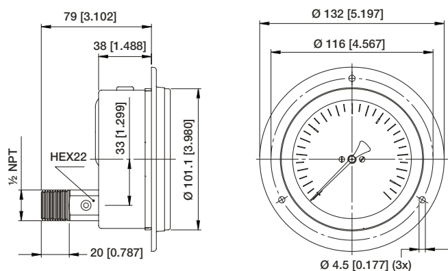
100mm SB 轴向连接 (XFF), 2500米
