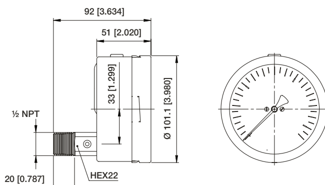
100mm SC 轴向连接, 2500米
