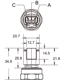
DS - Deutsch® DTM04-3P
