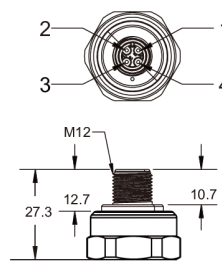
EX/RX/GX/LX(金属螺纹)
