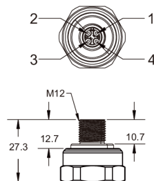
EW/RW/GW/LW(塑料螺纹)
