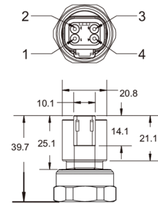
DU - Deutsch® DT04-4P
