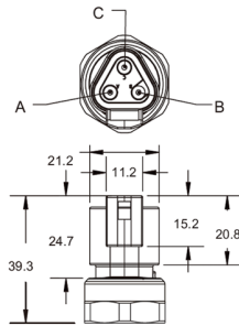
DT - Deutsch® DT04-3P
